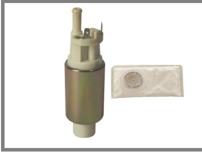
Yakıt Pompası Süzgeçli Fuel Pump With Filter 5,0 Bar UNIVERSAL - SLX - TEMPRA - TIPO 1.6IE - DKS
